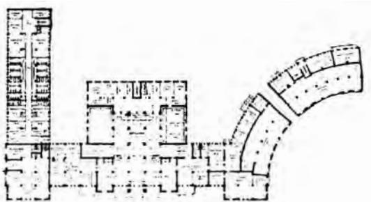
III премия, проект под девизом «Аист», общий вид, план 1 этажа, перспектива площадей Б. Л. Бородавкин, А. Н. Васильев, Н. А. Семенцов и др., консультант Е. А. Лымарь
