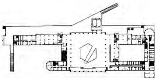
Аэропорт «Борисполь». Архитт. А. В. Добровольский, А. И. Малиновский, Д. П. Попенко, 1965
