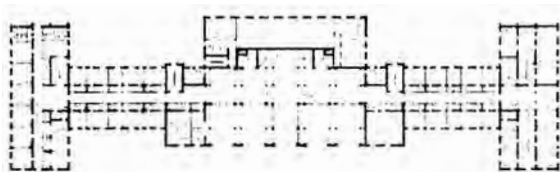
IV премия, проект под девизом «Киев», общий вид, план 2 этажа. Архит. М. И. Брусиловский
