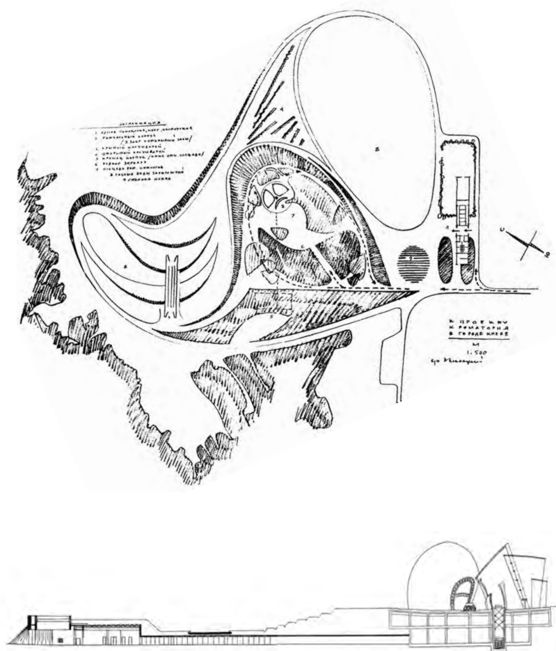
Эскизный генплан мемориального комплекса Парк Памяти, подземная коммуникация между крематорием и Залами прощания, разрез, 1968
