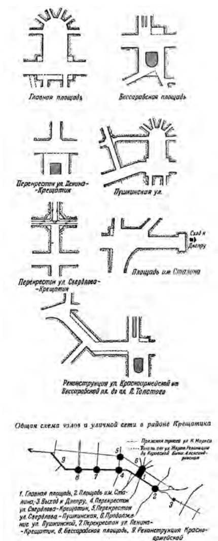
Схемы основных узлов Крещатика, составленные А. В. Власовым по материалам I конкурса
