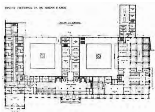
I премия, проект гостиницы под девизом «Треугольник в круге», 1939
