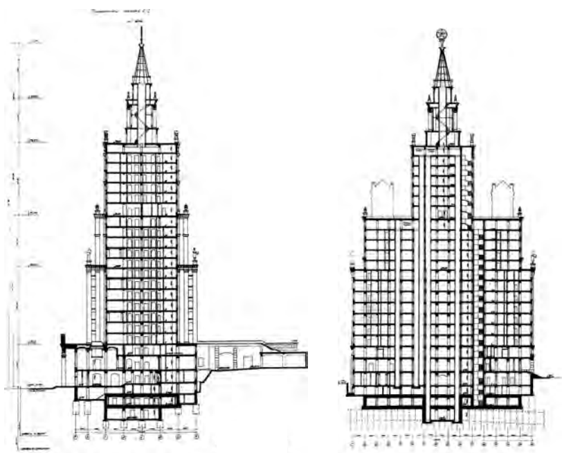
Гостиница «Москва». Боковой фасад, разрезы, вариант 1959
