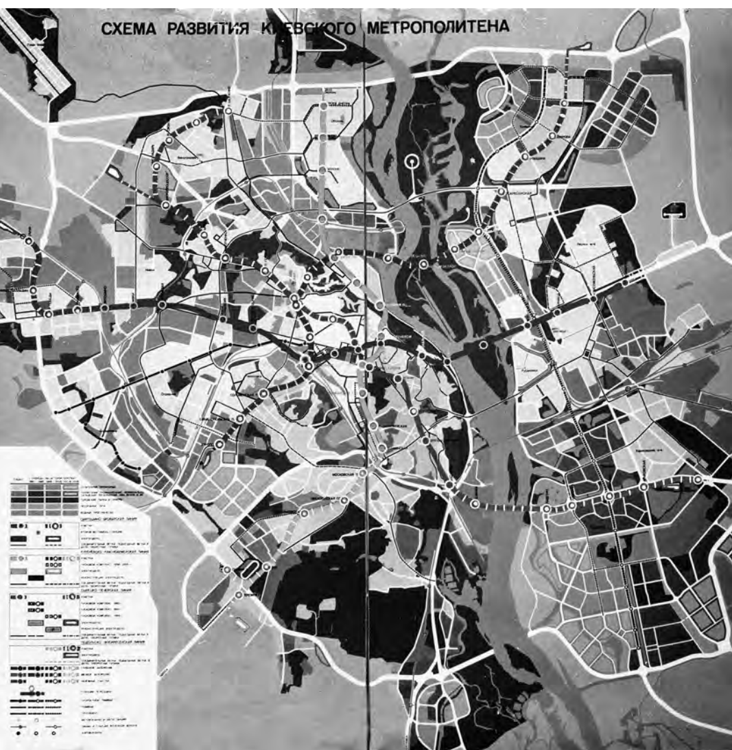
Схема развития киевского метрополитена. Инженеры И. Л. Казимиров, Я. Б. Левитан, 1980-е
