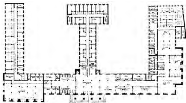
Упремия, проект под девизом «Родине», общий вид, план 1 этажа
