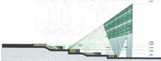
Боковий фасад М 1:100
