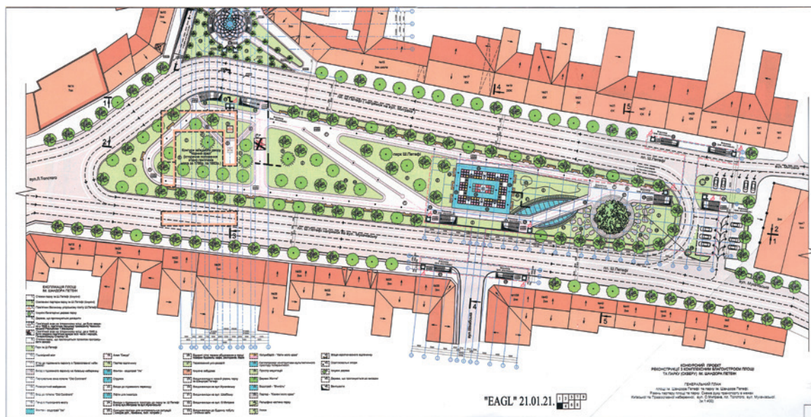
Ескізний проект реконструкції площі Шандора Петефі: план, розрізи, благоустрій
