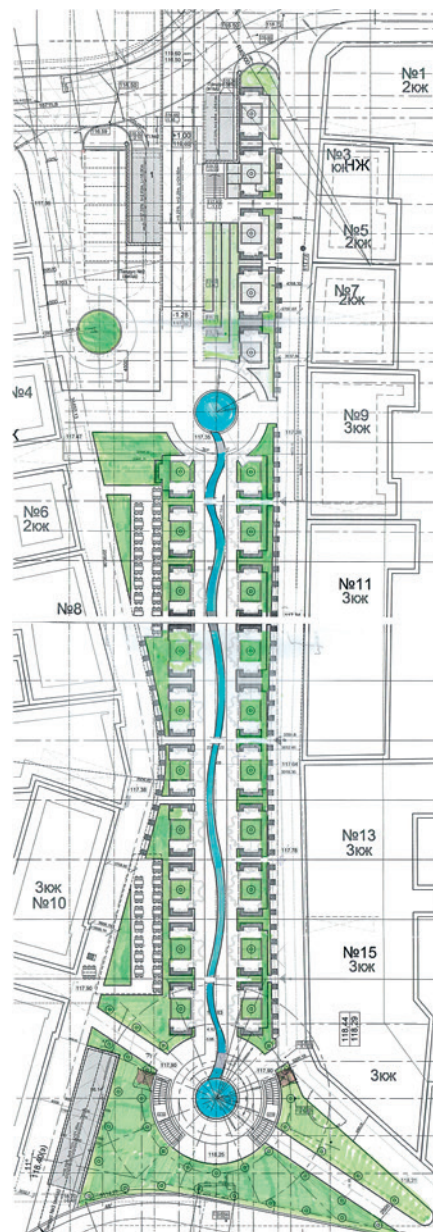
Ситуаційний генплан і партер площі Шандора Петефі, архіт. Я. Віг, 2017
