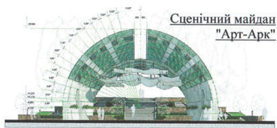
Головний фасад в вісях А-Г зі сторони Майдану народних свят та зустрічей М 1:100
