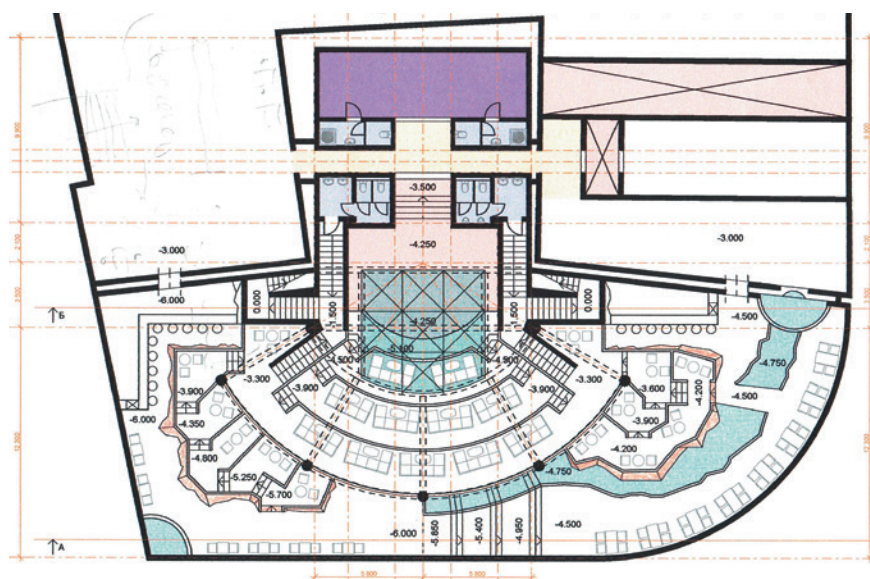
План підземного поверху на вігм. -3,3
