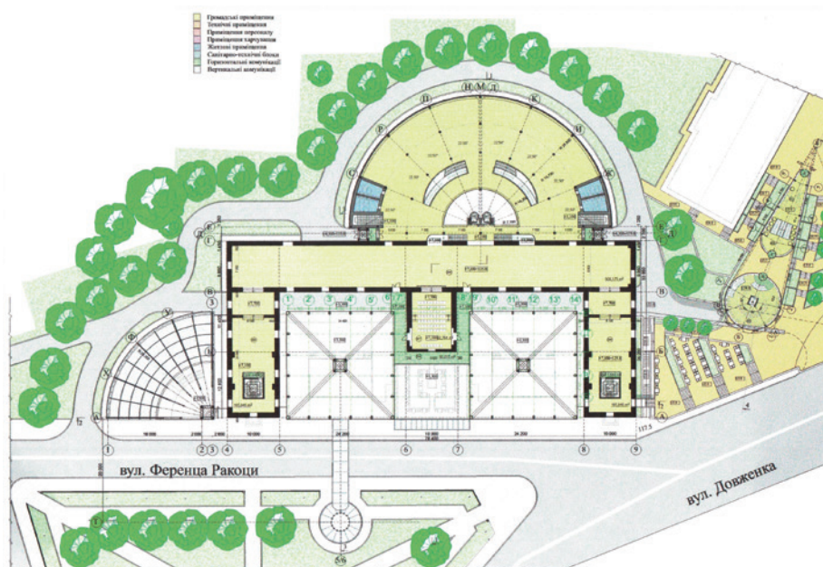
План другого поверху на відм. +7.100=125.8 М 1:200
